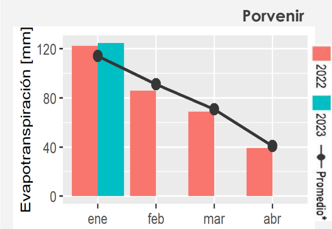
Figura 13. Evapotranspiración acumulada mensual para dos localidades de la Zona Austral entre enero y abril de 2022, enero de 2023 y promedio. Datos: DMC. *Promedio obtenido en 8 años de datos.
