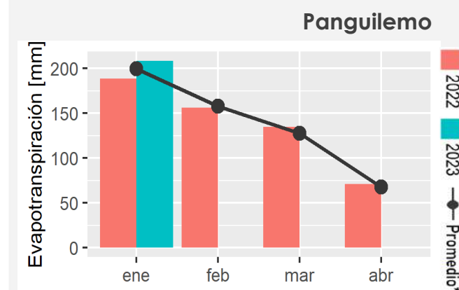
Figura 11. Evapotranspiración acumulada mensual para dos localidades de la Zona Central entre enero y abril de 2022, enero de 2023 y promedio. Datos: DMC. *Promedio obtenido en al menos 3 años de datos.
